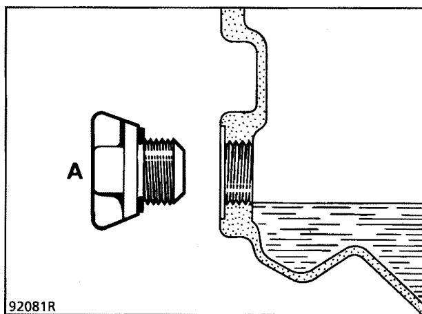
Пробка (А) без щупа
